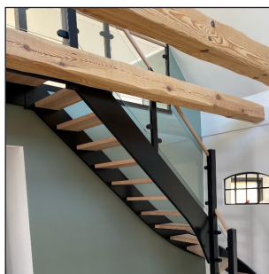
Glas monteret med klembeslag
