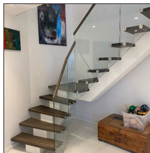
Glas monteret med adaptore
