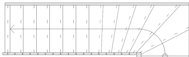
T-11 kvartsvingstrappe
